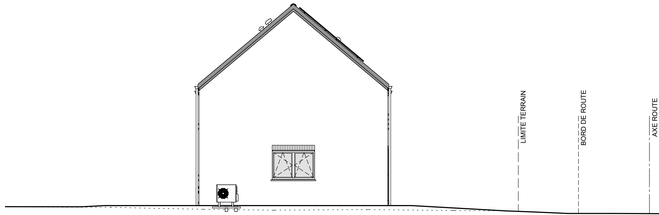
PIGNON GAUCHE
