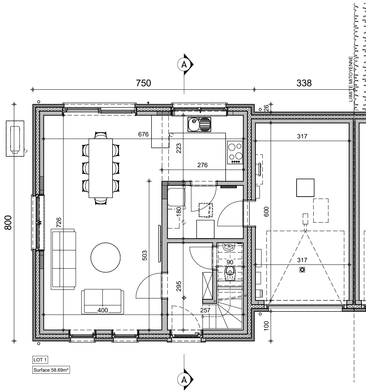
REZ-DE-CHAUSSEE
