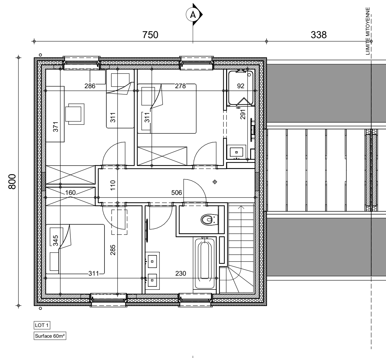
ETAGE
